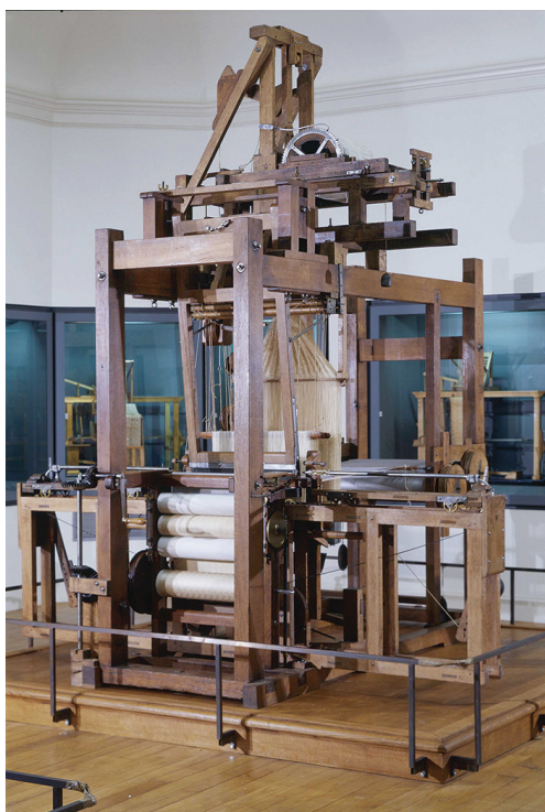
Métier à tisser les étoffes façonnées de Vaucanson, 1746. Inventaire n°: 00017-0001. Jacques de Vaucanson, 1709-1782, inventeur et mécanicien, France. Textile © Musée des arts et métiers-Cnam/photo Sylvain Pelly
